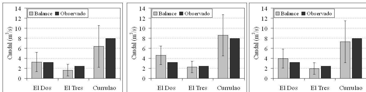
Figura 6. Caudales medios e incertidumbres asociadas a la aplicación del método del balance hidrológico utilizando el método de cálculo de la evapotranspiración de (a) Cenicafé-Budyko, (b) Turc, y (c) Choudhury.
