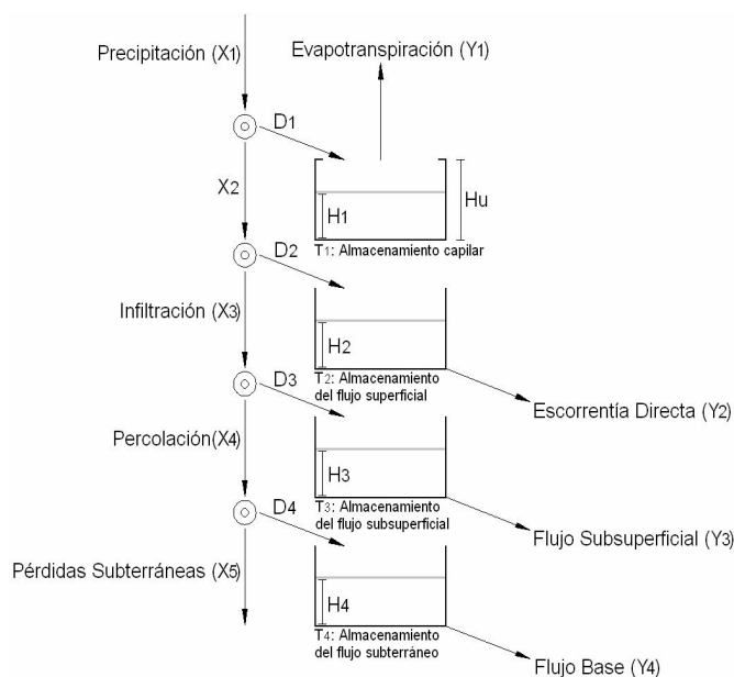
Figura 3. Esquema conceptual del modelo de tanques.
