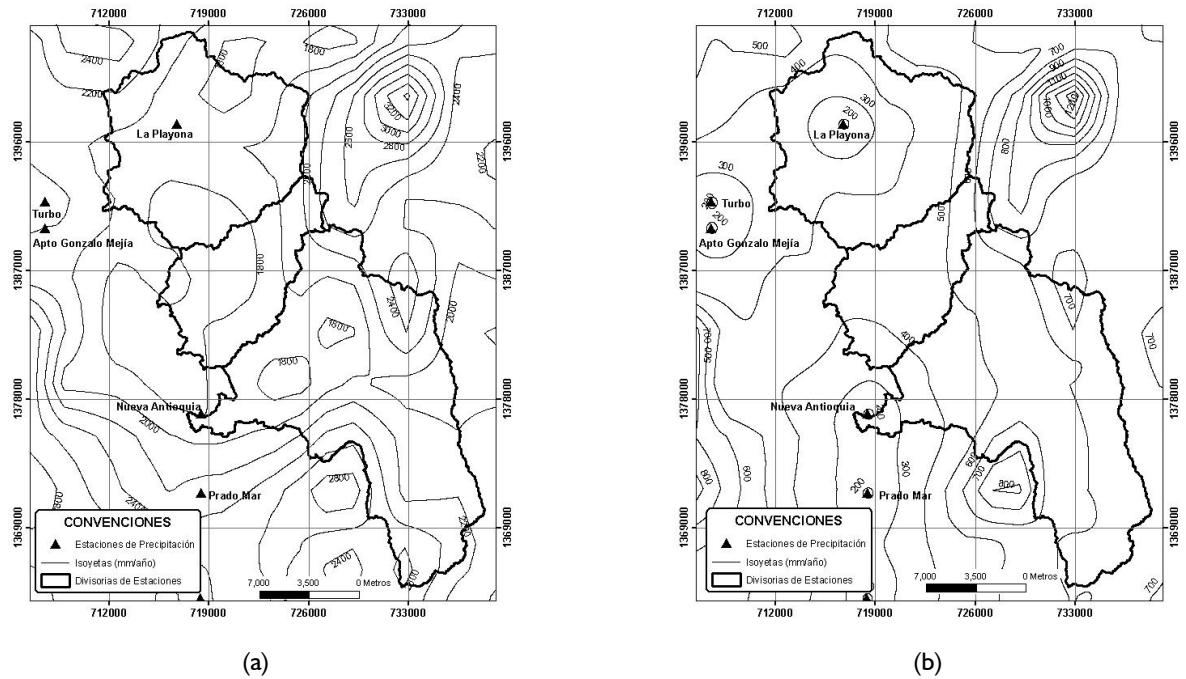
Figura 4. Campo de precipitación media multianual (a) e incertidumbre asociada (b), utilizando el método KDE con mapa de derivas de la TRMM.
