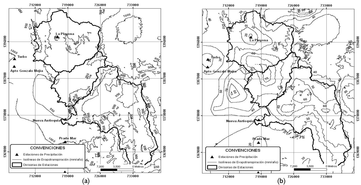
Figura 5. Mapa de evapotranspiración real media multianual por el método de Turc (a) y su incertidumbre asociada (b).
