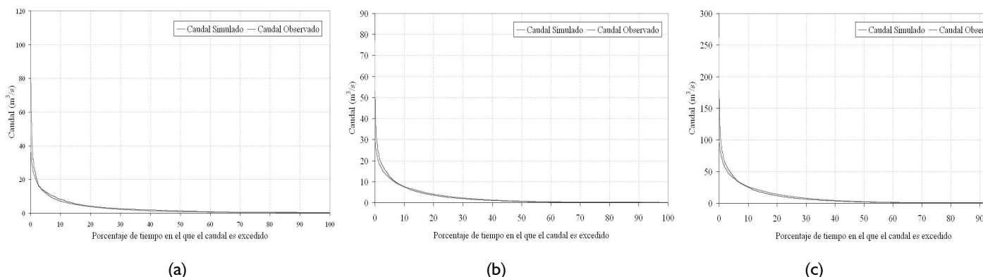
Figura 8. Curvas de duración de las series simuladas y observadas en las estaciones (a) El Dos, (b) El Tres y (c) Currulao.
